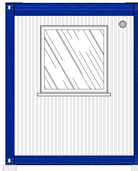
ELEWACJA TYLNA
